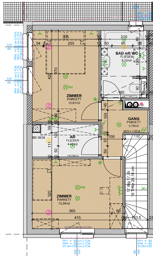
1. Obergeschoss
