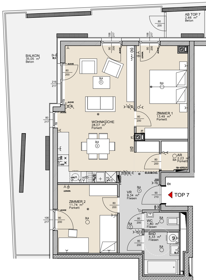
ÜBERSICHT 1. OBERGESCHOSS
