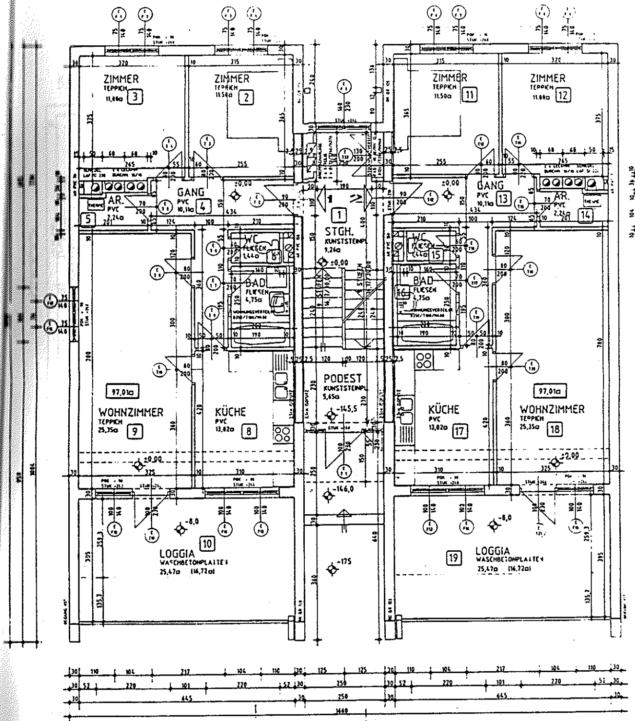
ERDGESCHOSS
